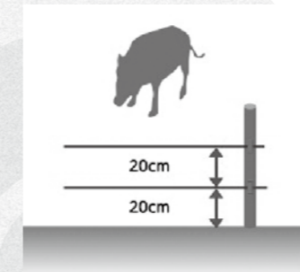
イノシシ用電気柵の設置間隔
