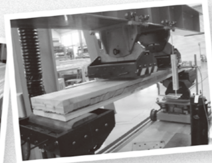
曲げたときの強度性能の試験
