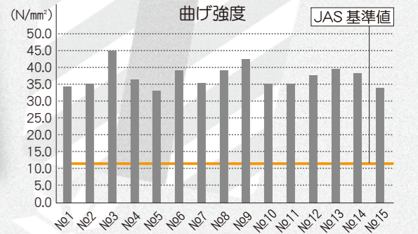
曲げたときの強度性能の試験
