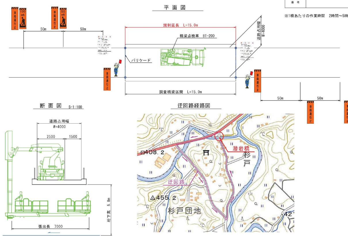
交通規制計画図（規制パターンB） 車両通行止め規制（新市赤名線：潜岩橋）
